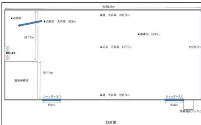
1階平面図
