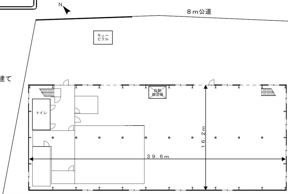
1階平面図
