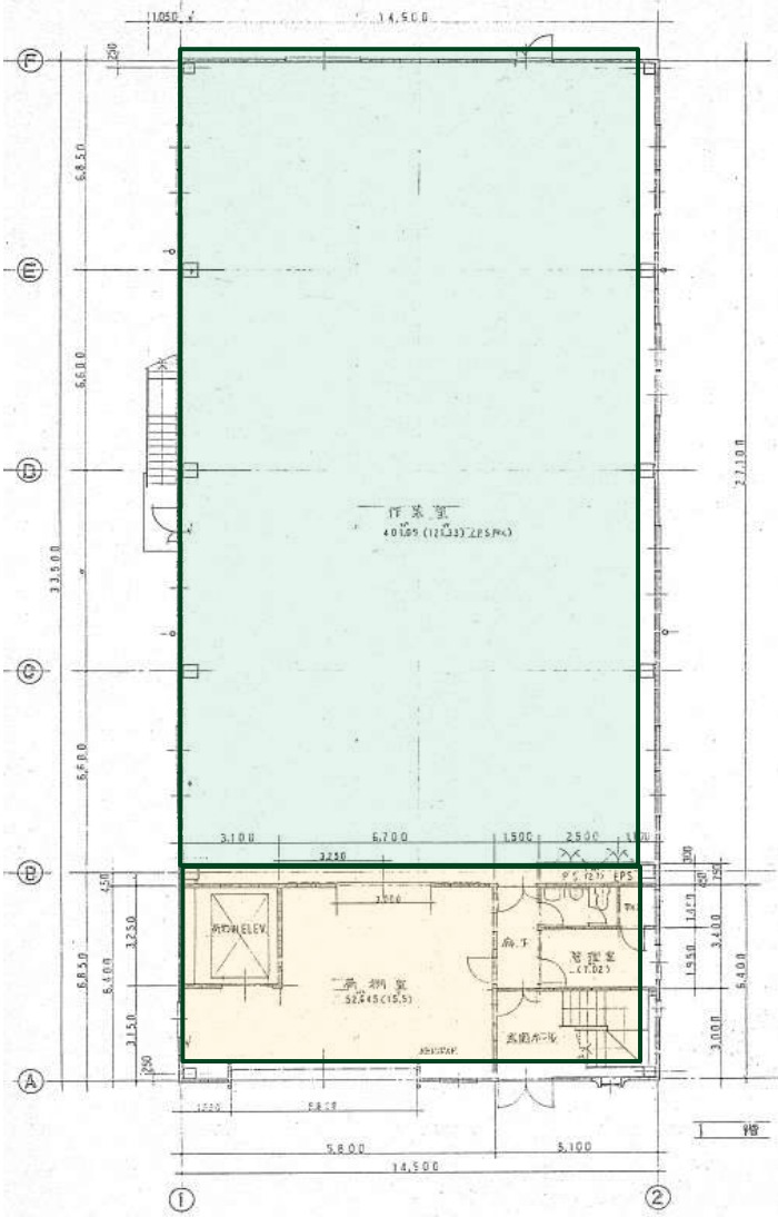
1階平面図
