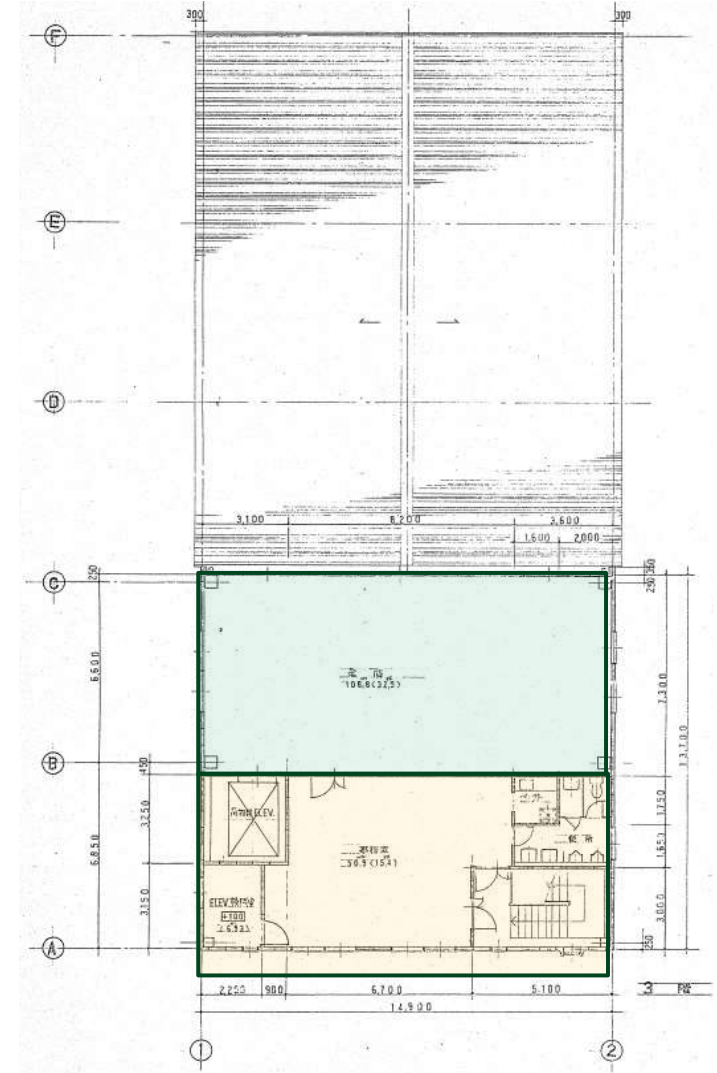
3階平面図
