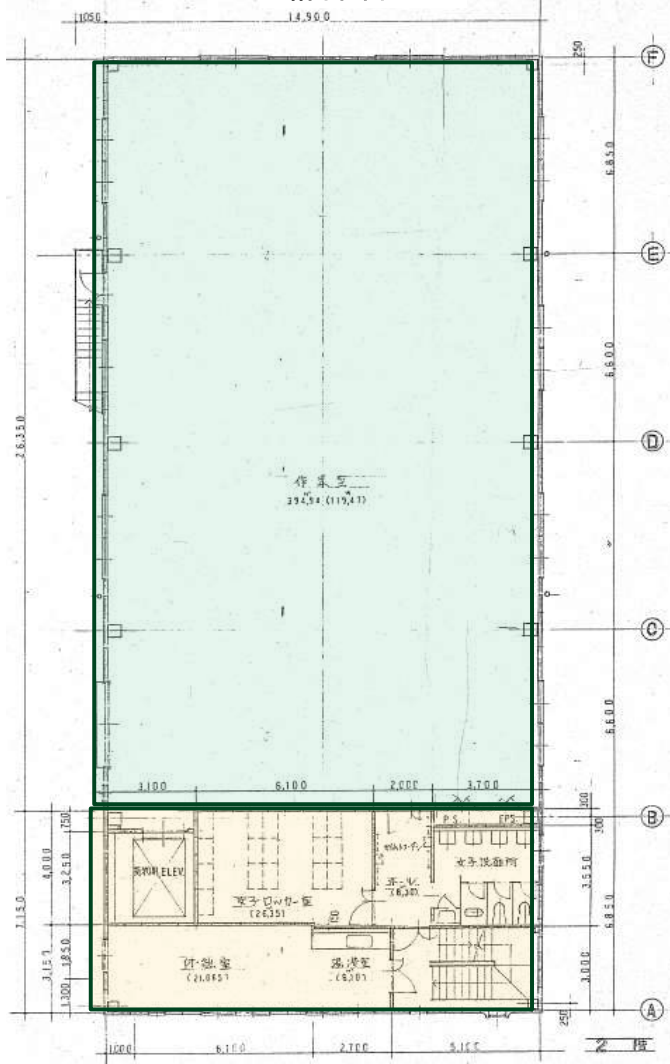
2階平面図
